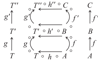
Рис. 3. Пример g, g' -транзактированной, f, f' -клонированной структуры обов
