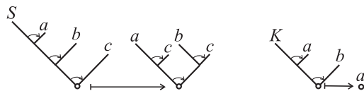
Рис. 1. Характеристики комбинаторов S и K
