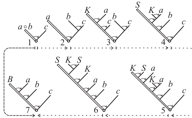
Рис. 2. Характеристика комбинатора композиции B и выращивание дерева вычислений для B , пользуясь деревьями для комбинаторов S и K . (Пояснение. Переход от композиции a \circ b (дерево 1) к представляющему комбинатору B (дерево 7) получается при обходе против часовой стрелки. Для этого потребуется шесть шагов, если имеются только деревья вычислений для S и K )
