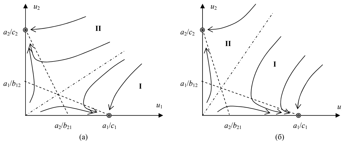
Рис. 2. Изменение фазовых траекторий в обществе восточного типа при уменьшении отношения c_1/b_{21} в уравнении (1) (см. пояснения в тексте): а) начальное состояние; б) конечное состояние
