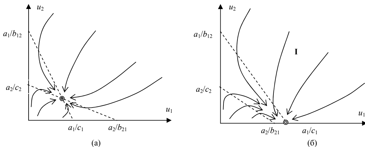
Рис. 3. Изменение фазовых траекторий в обществе западного типа при уменьшении отношения c_1/b_{21} в уравнении (1) (см. пояснения в тексте): а) начальное состояние; б) конечное состояние
