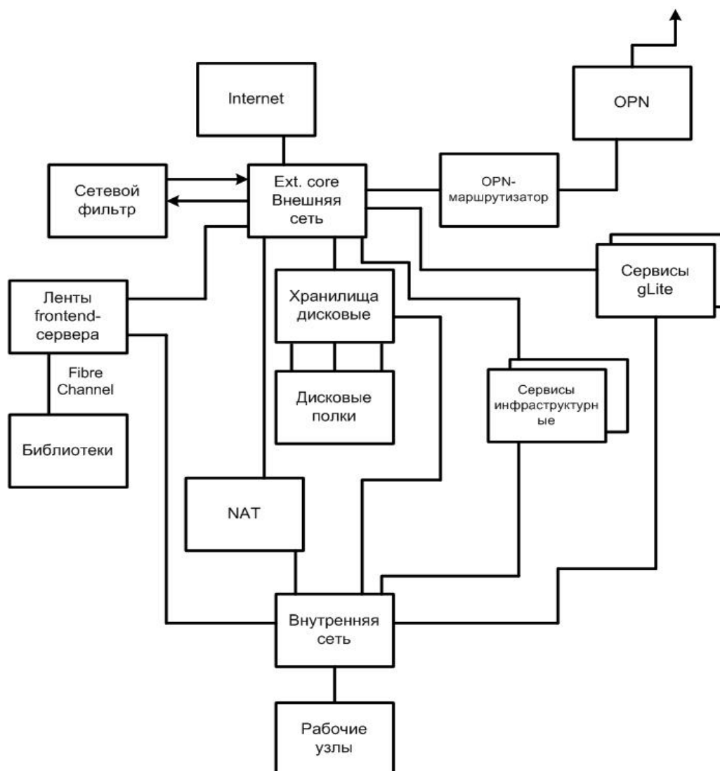
Рис. 6. Схема структуры центра Tier-1 НИЦ «КИ»
