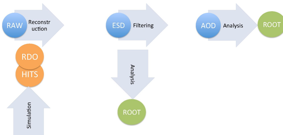
Рис. 2. Форматы данных и стадии их обработки в ALICE
