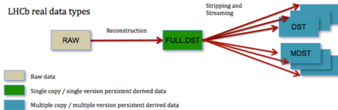
Рис. 4. Модель обработки данных LHCb
