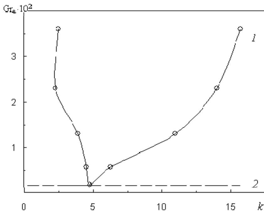
Рис. 2 Область устойчивости двумерных стационарных пространственно-периодических вихревых структур ЭК-течения слабопроводящей жидкости с униполярной инжекционной проводимостью в плоскопараллельной системе электродов
