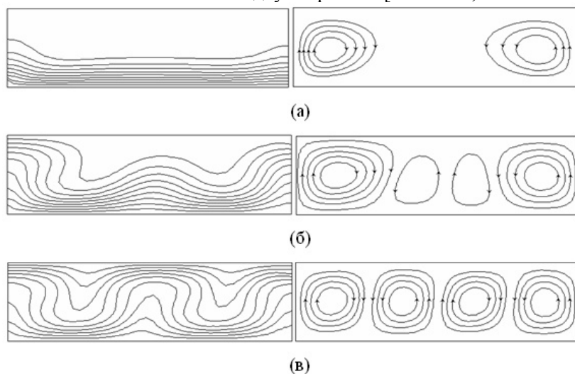
Рис. 1 Изолинии объёмной плотности зарядов (слева) и линии тока (справа)
